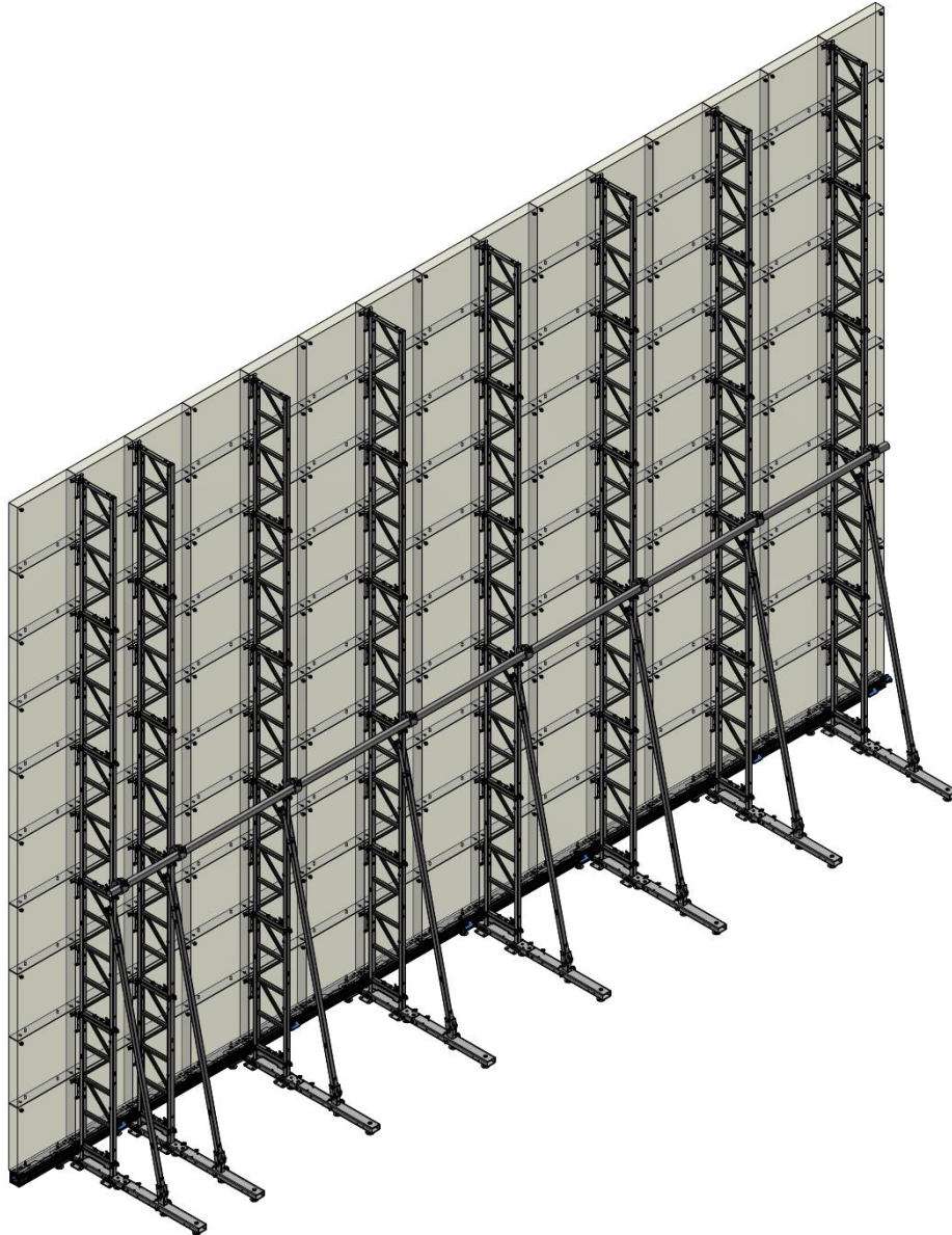
Abbildung 48 Serie DB 15x10 isometrische Ansicht
