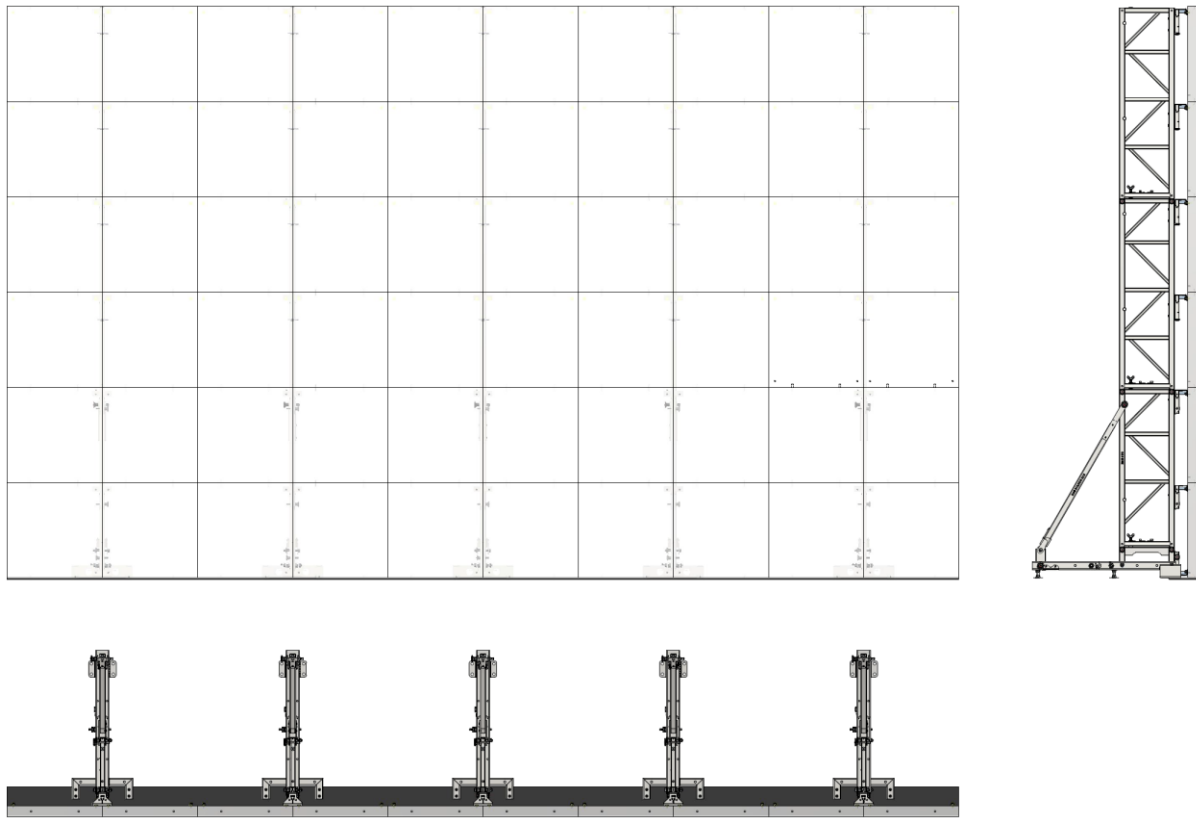
Abbildung 53 AURA 10x6 Ansichten
