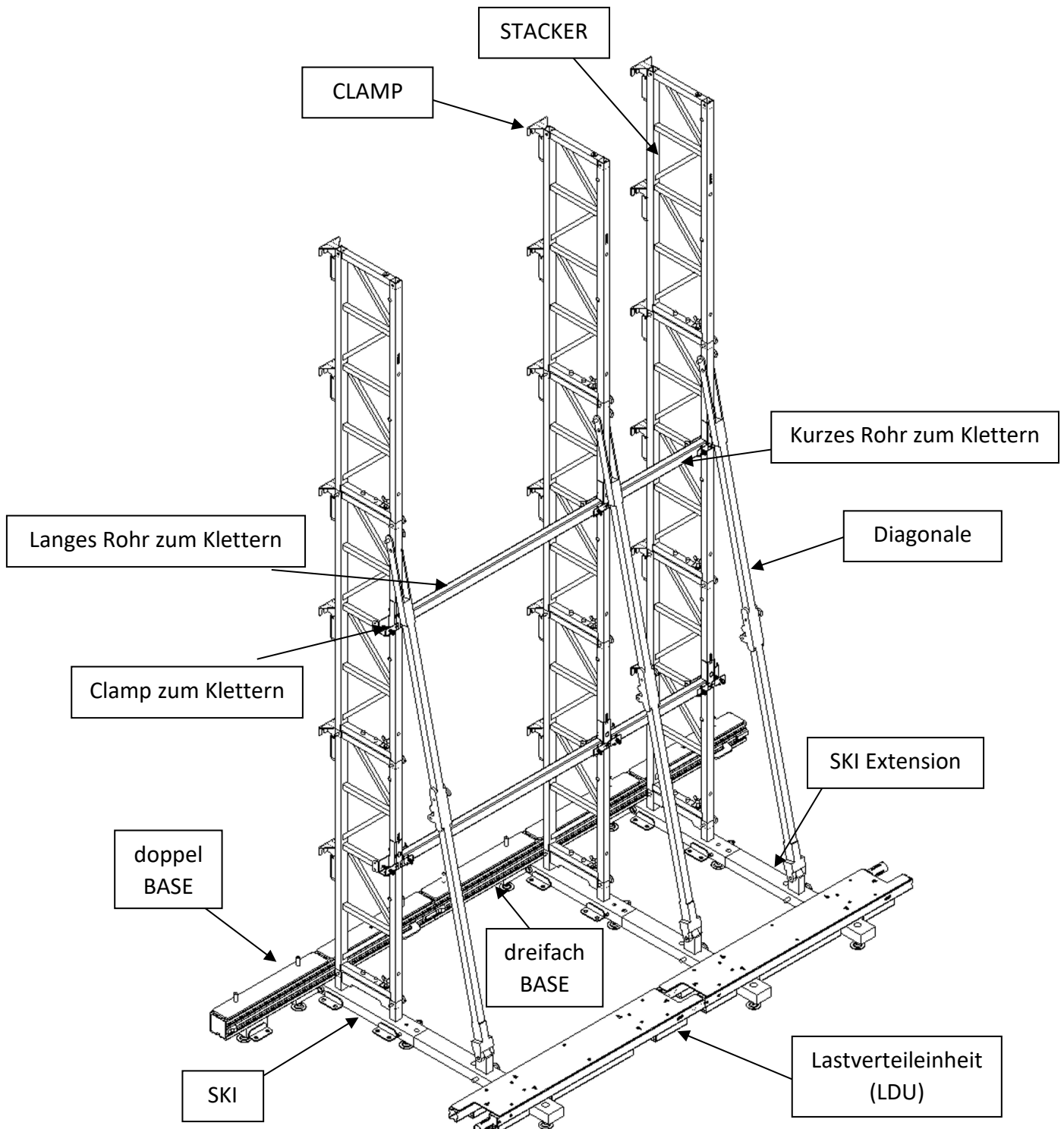
Abbildung 3 Beispielhafte Übersicht der PLS-Komponenten ohne LED-Module
