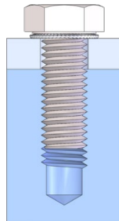
Abbildung 7 Korrekte Ausrichtung der Schnorr-Sicherheitsunterlegscheibe (Foto von Schnorr)
