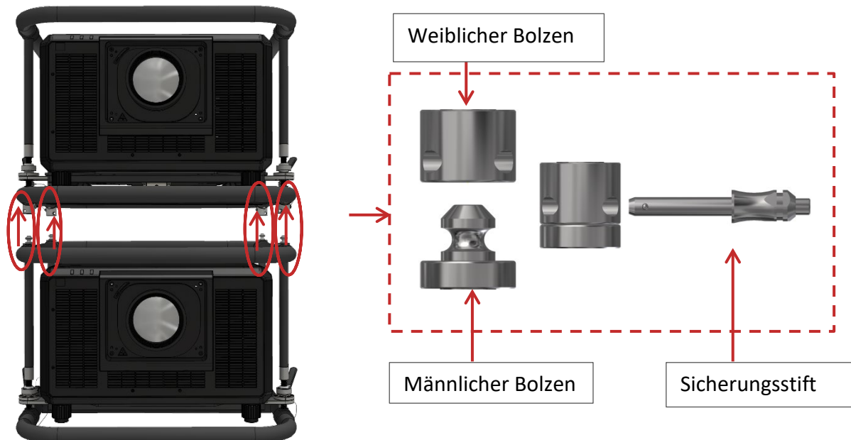
Abbildung 12 Stapeln von Rahmen
