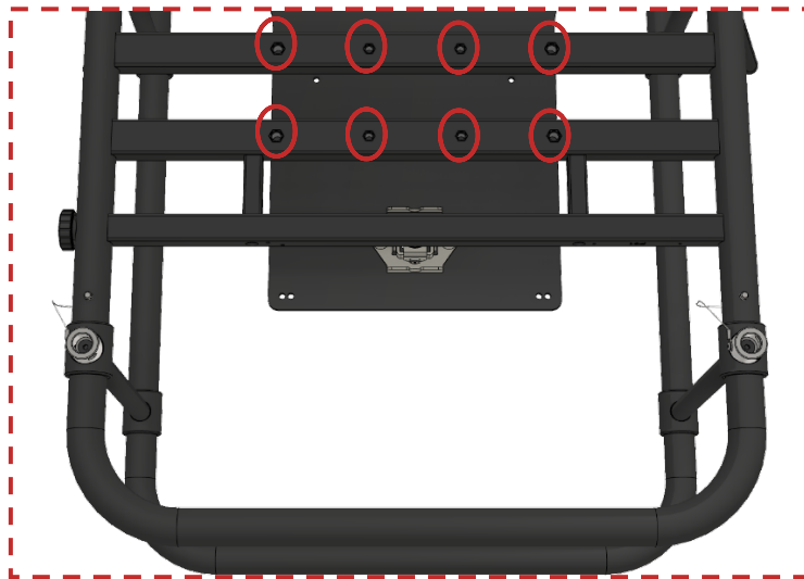
Abbildung 17 Kontrolle der Montagegewinde an der Unterseite
