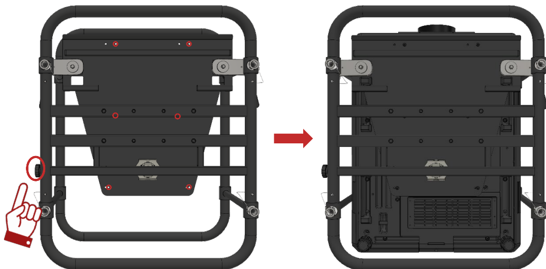
Abbildung 4 Montage des Projektors im Rahmen
