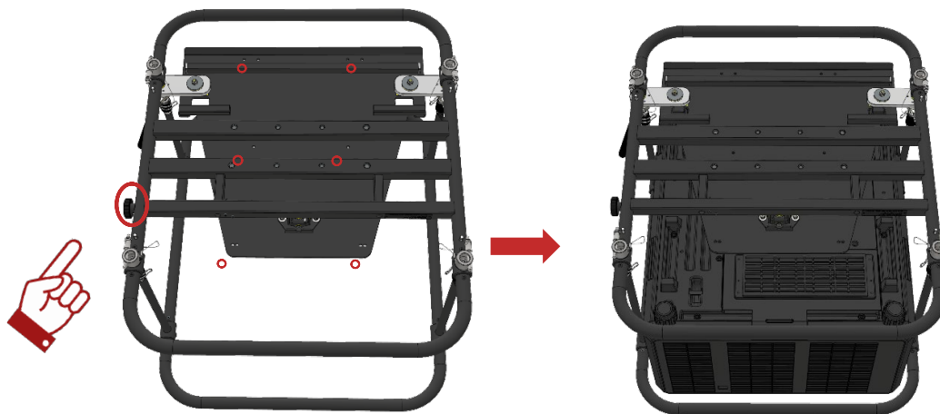
Abbildung 4 Montage des Projektors im Rahmen
