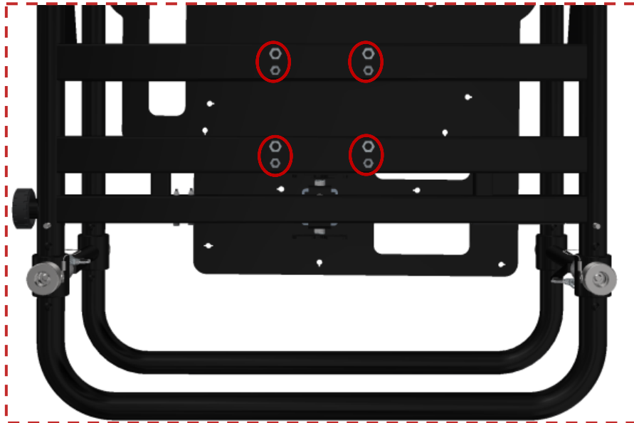
Abbildung 25 Kontrolle der Montagegewinde an der Unterseite
