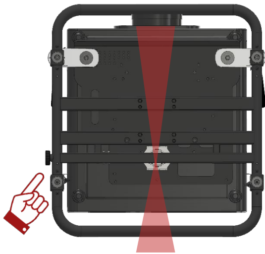
Abbildung 19 Einstellung: Yaw
