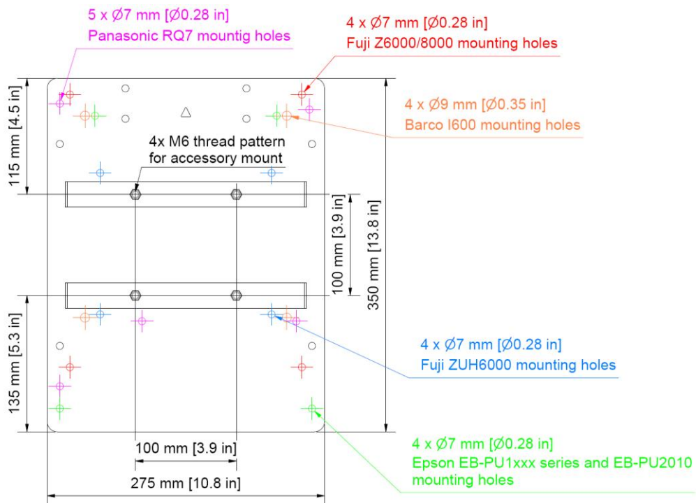
Abbildung 8 Beispiel-Befestigungslöcher für verschiedene Projektoren
