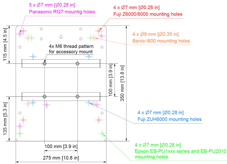
Abbildung 13 Projektor-Befestigungslöcher
