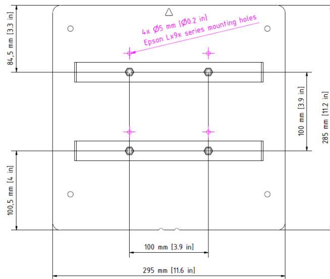
Abbildung 9 Befestigungslöcher für ECO Frame E1.0
