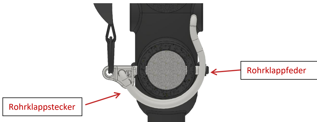
Abbildung 11 Querschnittsansicht eines ordnungsgemäß geschlossenen Rohrklappsteckers
