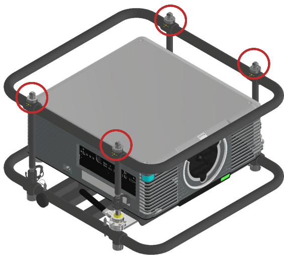
Abbildung 26 Stapelpunkte Oberseite
