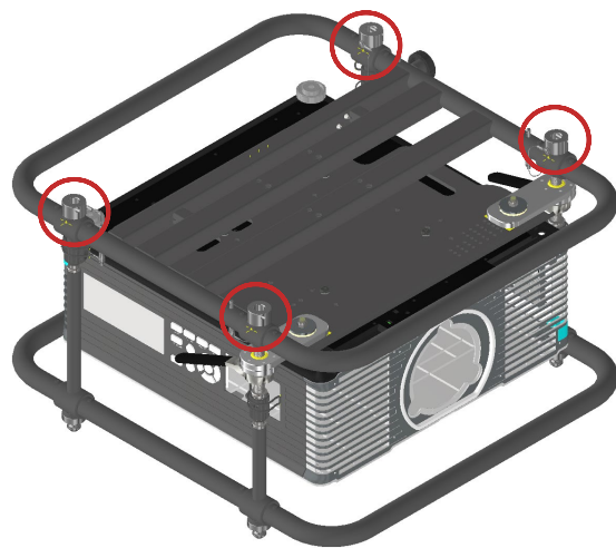
Abbildung 27 Stapelpunkte Unterseite
