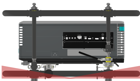
Abbildung 16 Einstellung: Pitch
