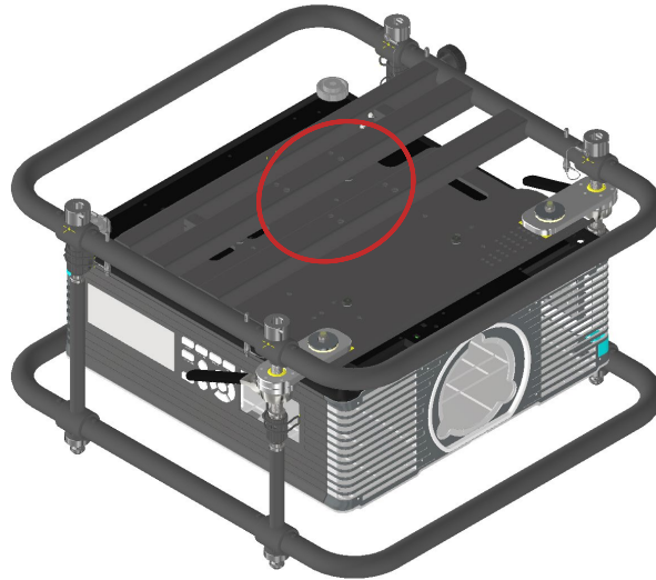
Abbildung 19 Gewinde an der Unterseite des Rahmens
