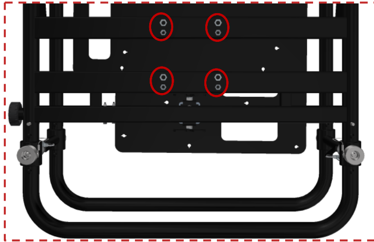
Abbildung 23 Kontrolle der Montagegewinde an der Unterseite
