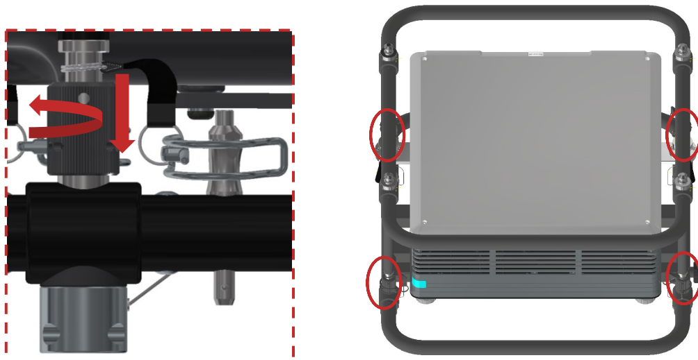
Abbildung 12 Festziehen der vier Befestigungsmuttern
