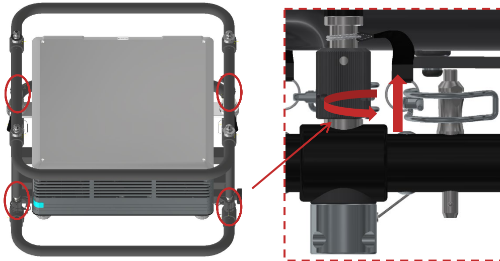
Abbildung 9 Lösen der vier Befestigungsmuttern
