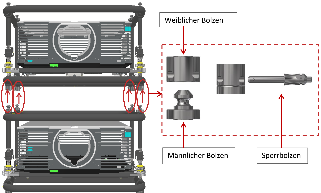
Abbildung 18 Stapeln von Rahmen
