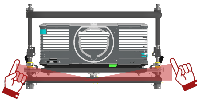
Abbildung 15 Einstellung: Roll
