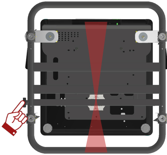
Abbildung 17 Einstellung: Yaw
