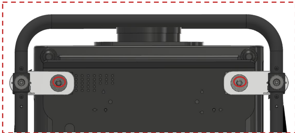
Abbildung 26 Muttern auf der vorderen Unterseite, die mit rotem Wachs versiegelt sind
